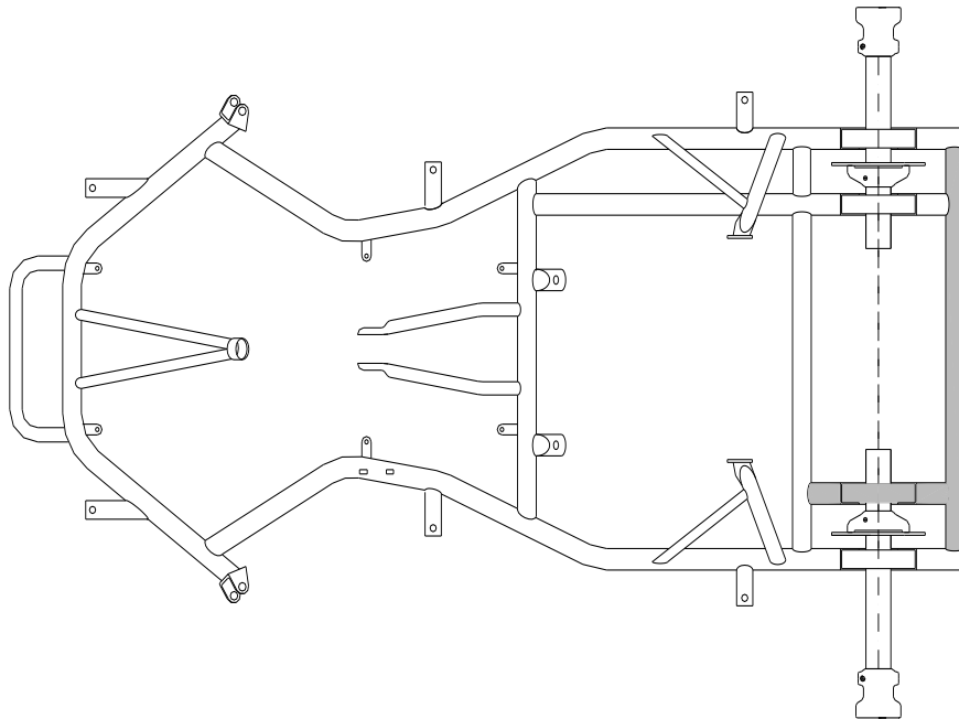
Figure 5 Châssis avec essieu arrière coupé en deux pièces, roulements à l'extrémité, avec addition de tubes C1 et C2 au châssis
