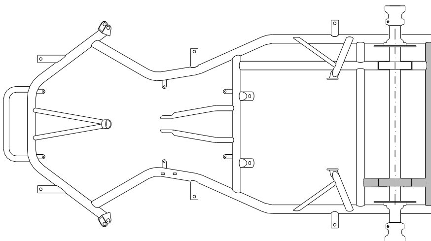
Figure 6 Châssis avec essieu arrière entier fixes, moyeux de rue avec roulements, et addition de tubes C1 et C2
