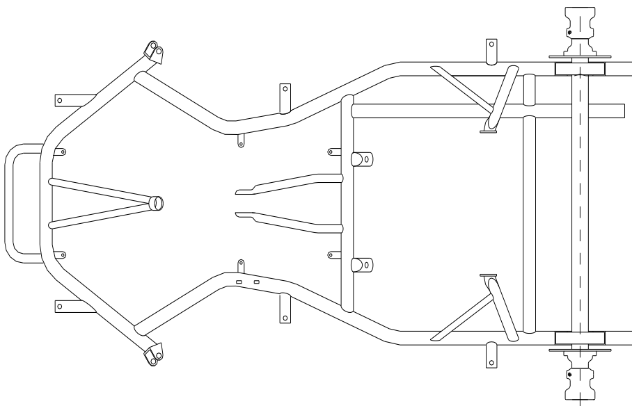
Figure 4 Châssis avec essieu arrière entier fixes, moyeux de roue avec roulements, sans addition de tubes C1 et C2
